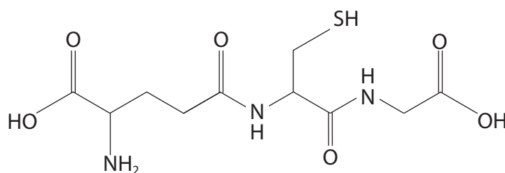
glutathione
